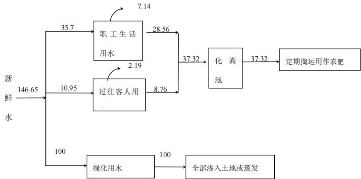
图 2-5 建设项目水平衡图 （单位：m³/a）
