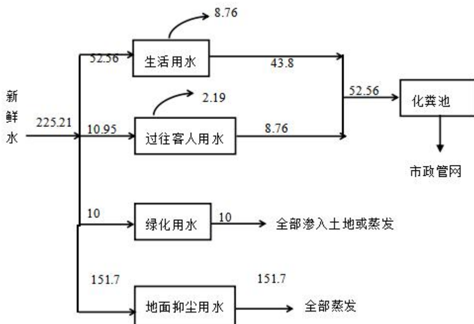
图 2-5 建设项目水平衡图 (单位: m 3 /a)
